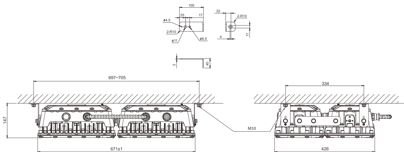
BR-TK-2-SUS316
